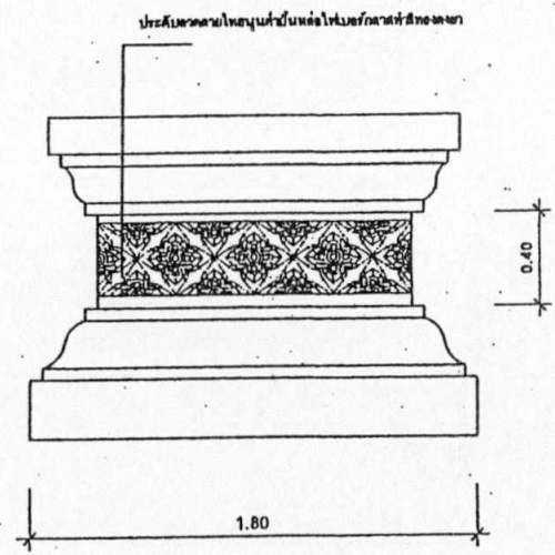
แบบขยายความ 7 มาตราส่วน 1 : 10
