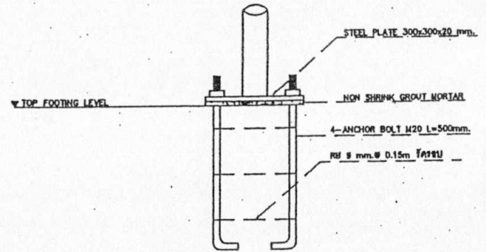
แบบขยายเพลา มาตราส่วน 1:130
