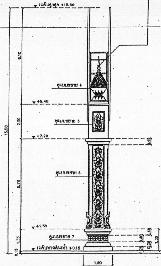
รูปคานข้าง
