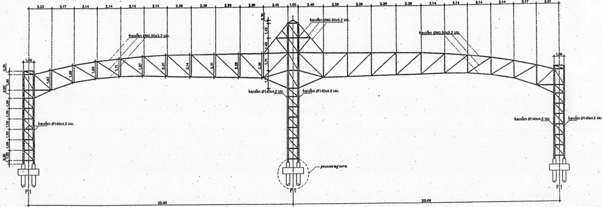
ชื่อยาว Truss1 ขนาดย่อ 1:150
