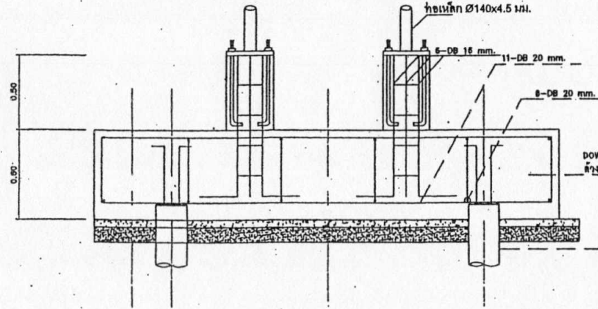
แบบขยายฐานราก F1 มาตราส่วน 1:125
