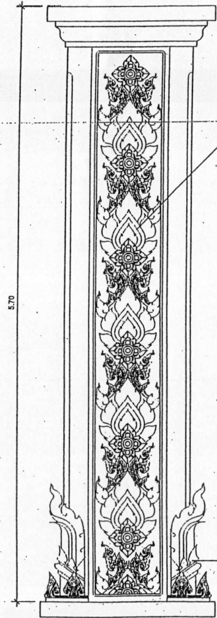
แบบขยายความ 6 มาตราส่วน 1 : 10
