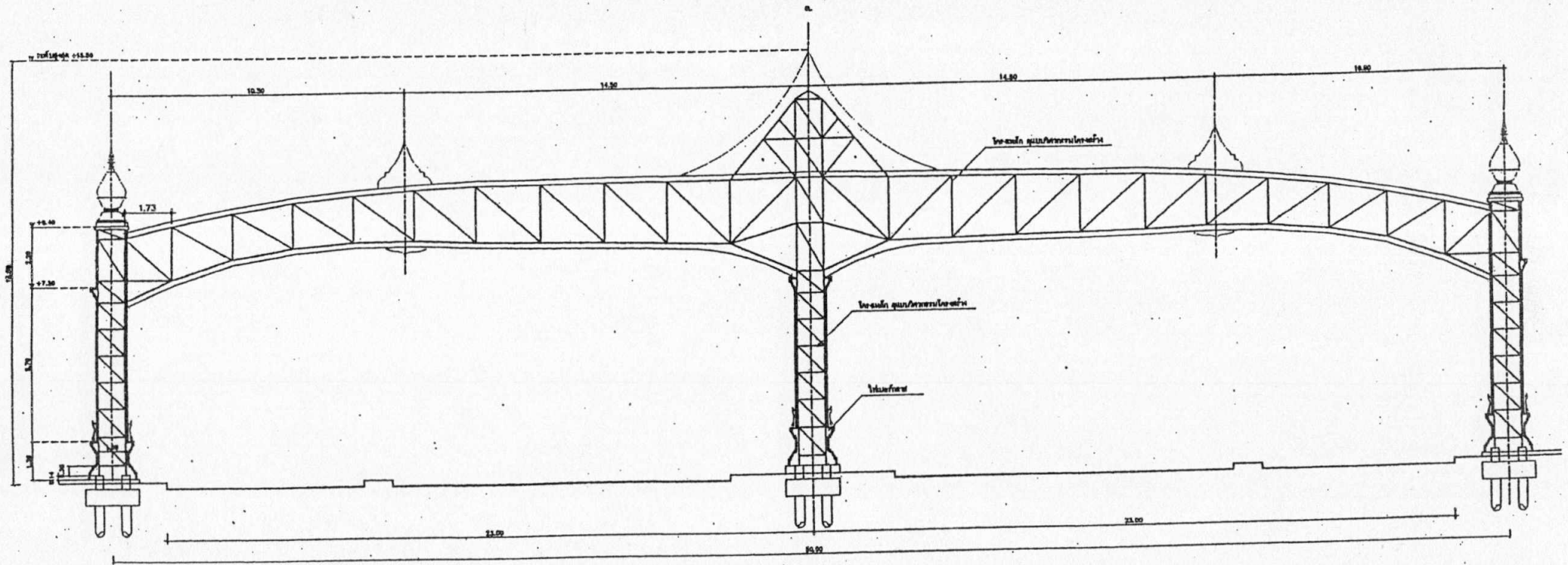
รูปตัด A-A ขนาด 1 : 100
